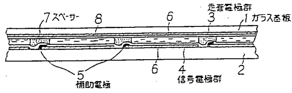
素子の部分断面図 第1図
